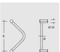
ES 21.300.4 ks, Ø 21 mm, Опори Ø 30 mm, разст. на закр. 300 mm
