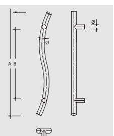
ES 21.400.5 sw, Ø 21 mm, Опори Ø 30 mm Дължина 500 mm, разст. на закр. 400 mm
