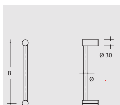
ES 21.300.4 gk, Ø 21 mm, Опори Ø 30 mm, разст. на закр. 300 mm
