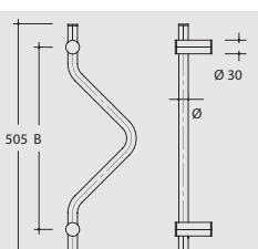
ES 21.400.5 sw, Ø 21 mm, Опори Ø 30 mm Дължина 500 mm, разст. на закр. 400 mm
